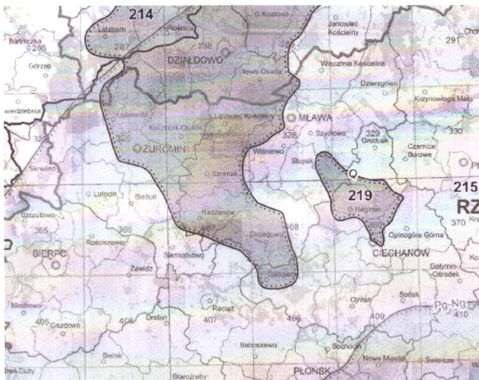
Ryc. 4. Usytuowanie Gminy Radzanów w otoczeniu GZWP
