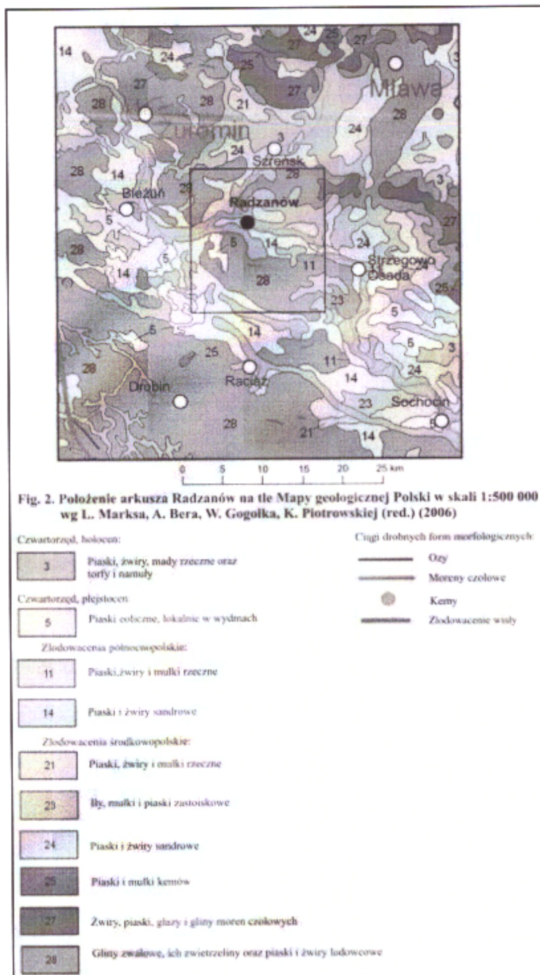
Ryc. 6. Geologia Gminy Radzanów Źródło: http://bazadata.pgi.gov.pl
