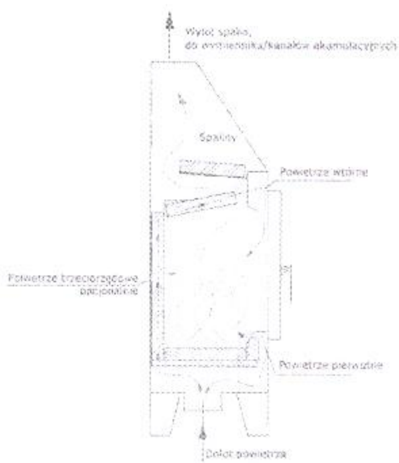
Rys. 1. Dystrybucja powietrza do spalania
